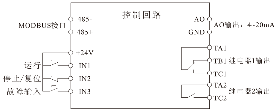
图 2.6 控制回路端子图
