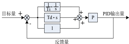
图 5-25 过程 PID 原理框图
