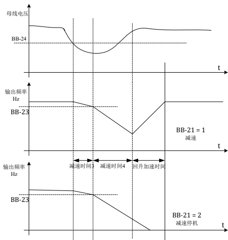
图 5-24 瞬时停电动作示意图
