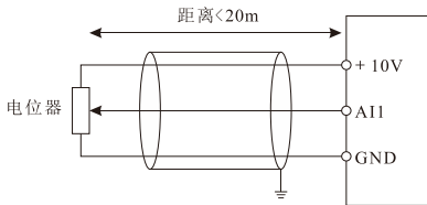
图 3-15 模拟量输入端子接线方式
