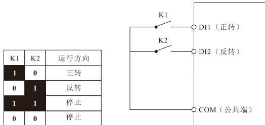
图 5-10 两线式模式 1
