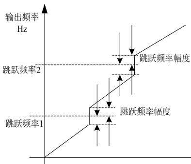
图 5-7 加减速过程中跳跃频率有效示意图
