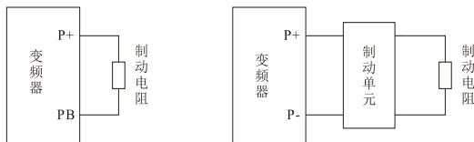
图 2-9 制动电阻连接示意图
