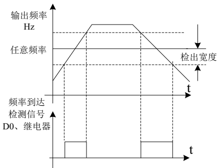
图 5-16 任意到达频率检测示意图
