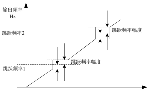
图 5-6 跳跃频率示意图
