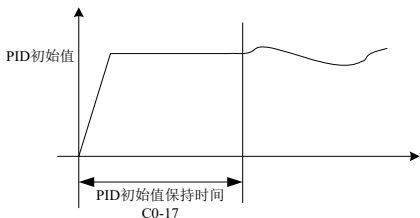
图 5-27 PID 初值功能示意图
