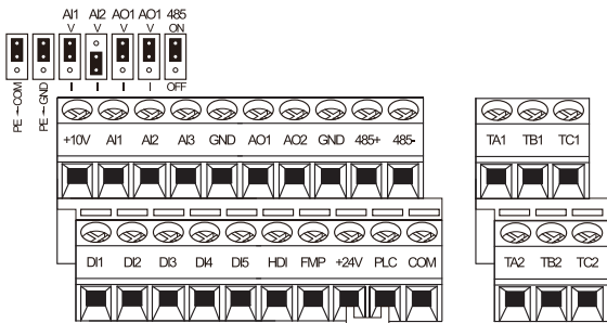
图 3-13 EM10 三相 4kW 以上控制回路端子图
