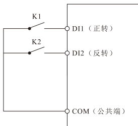
图 5-10 两线式模式 1
