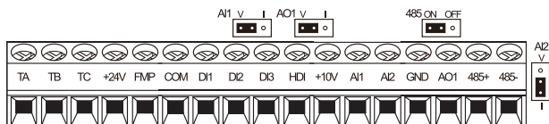
图 3-12 EM10 单相/三相 0.75 kW ~2.2kW 控制回路端子图
