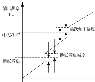
图 5-7 加减速过程中跳跃频率有效示意图
