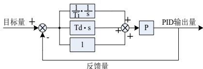
图 5-25 过程 PID 原理框图
