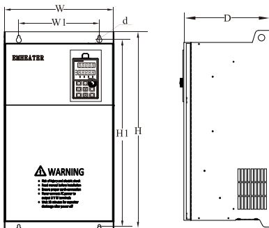
图 2-5 EM10 三相 30~500kW 壁挂安装尺寸图
