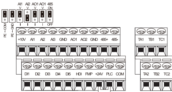
图 3-13 EM10 三相 4kW 以上控制回路端子图
