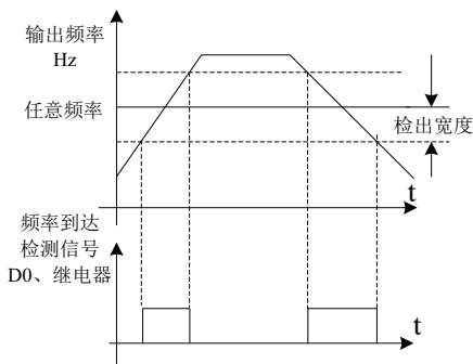
图 5-16 任意到达频率检测示意图
