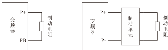
图 2-9 制动电阻连接示意图
