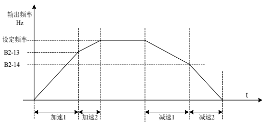
图 5-8 加减速时间切换示意图
