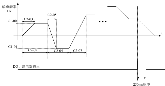
图 5-28 简易 PLC 示意图
