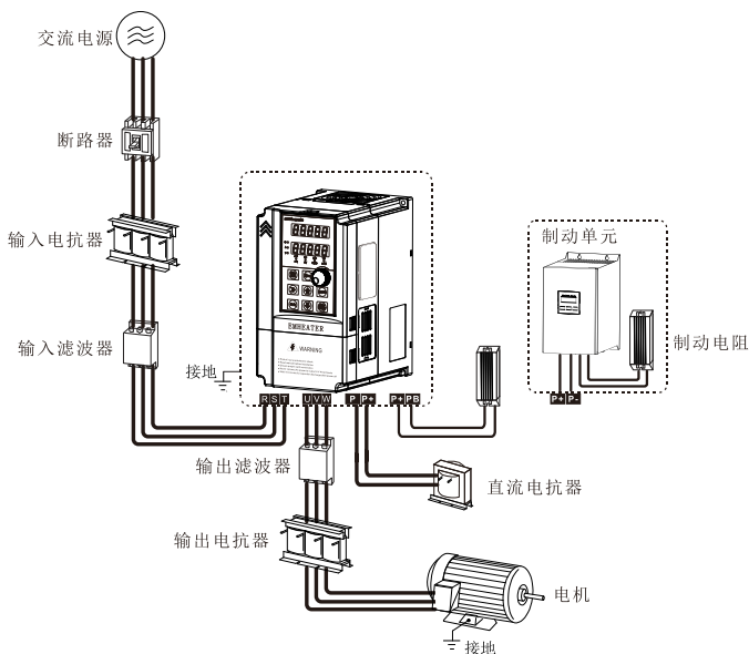
图 3-2 变频器外围设备连接图
