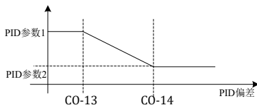
图 5-26 PID 参数切换
