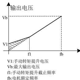
图 5-30 手动转矩提升示意图
