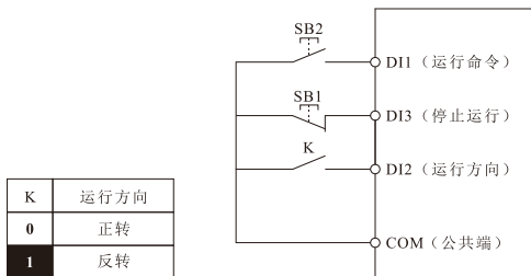
图 5-13 三线式控制模式 2
