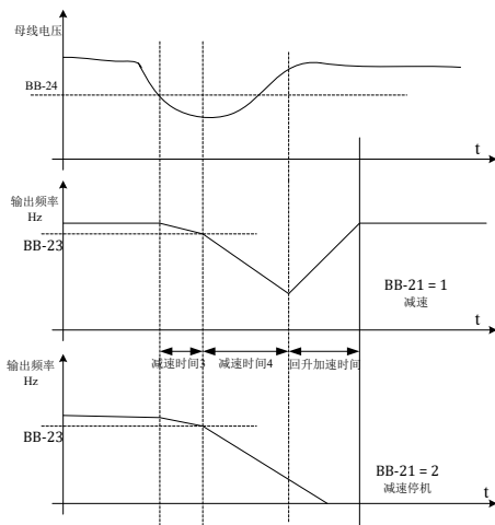
图 5-24 瞬时停电动作示意图
