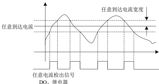
图 5-19 任意到达频率检测示意图
