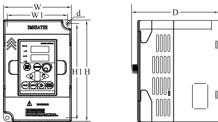
图 2-3 EM10 单相/三相 0.75~2.2kW 壁挂安装尺寸图
