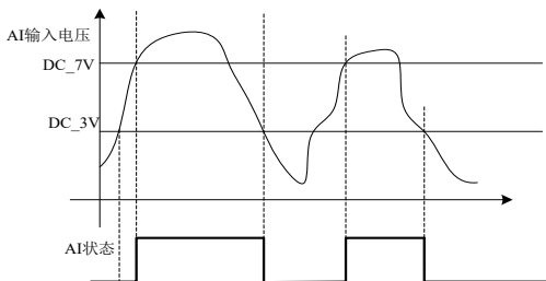
图 5-22 AI 端子有效状态判断
