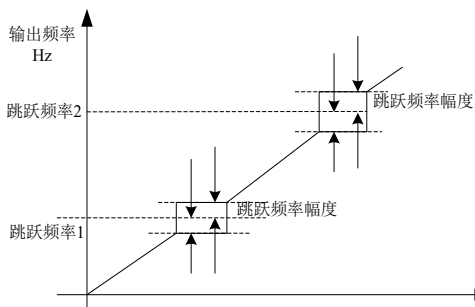
图 5-6 跳跃频率示意图
