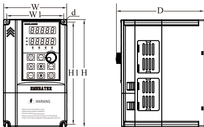
图 2-4 EM10 三相 4~22kW 壁挂安装尺寸图
