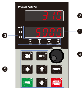
图 4-1 操作面板示意图
