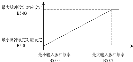
图 5-20 脉冲输入和设定值对应关系
