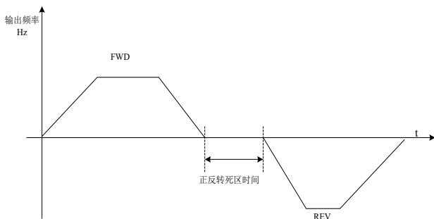
图 5-9 正反转死区时间示意图
