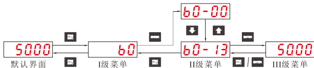
图 4-2 三级菜单操作流程图
