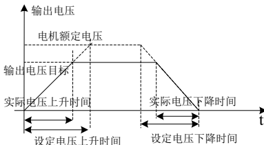
图 5-32 V/F 分离示意图
