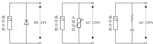
图 3-10 感性负载浪涌抑制器的应用示例
