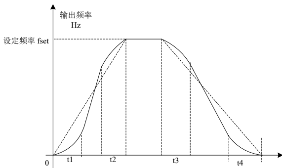
图 5-4 S 曲线加减速 A 示意图
