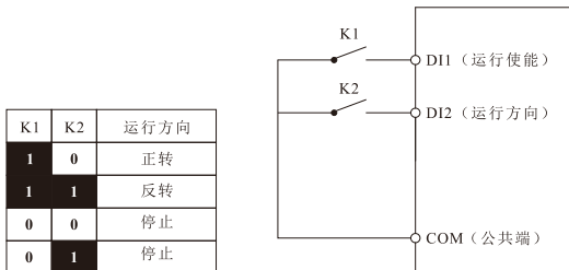
图 5-11 两线式模式 2
