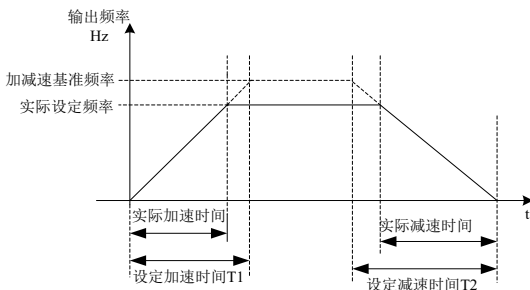
图 5-3 加减速时间示意图
