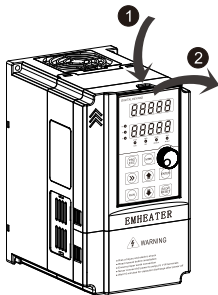
图 3-3 操作面板（键盘）的拆卸图
