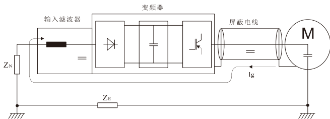
图 3-9 防传导辐射干扰接线示意图
