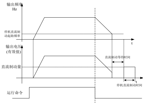
图 5-5 停机直流制动示意图
