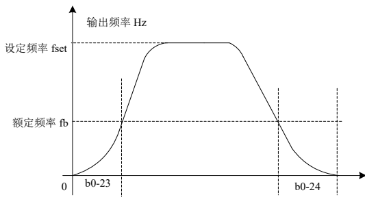
图 5-2 S 曲线加减速 B 示意图
