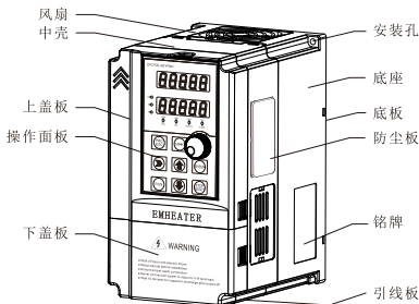
图 2-2 EM10 系列结构外型图
