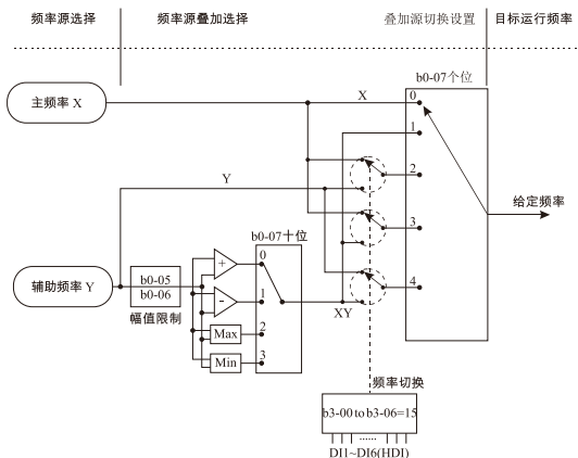
图5-1 目标频率设定示意图
