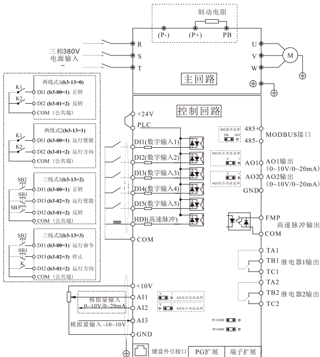
3-11 EM10 控制回路及主回路接线图
