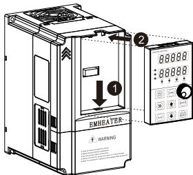
3-4 操作面板（键盘）的安装
