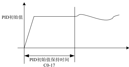
图 5-27 PID 初值功能示意图
