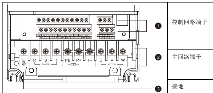
图 3-7 EM10 系列端子布局图示
