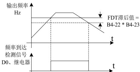
图 5-14 FDT 电平示意图
