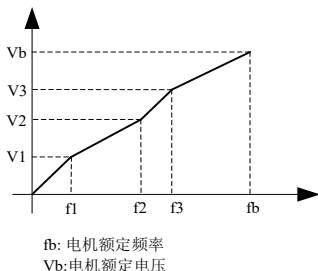
图 5-31 多点 V/F 曲线设定示意图
