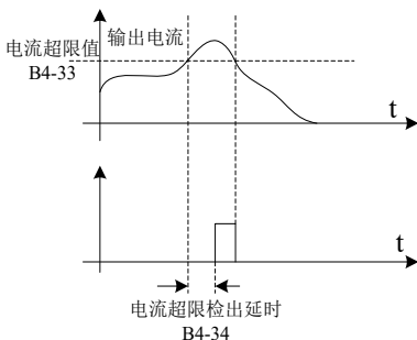
图 5-18 输出电流超限检测示意图
